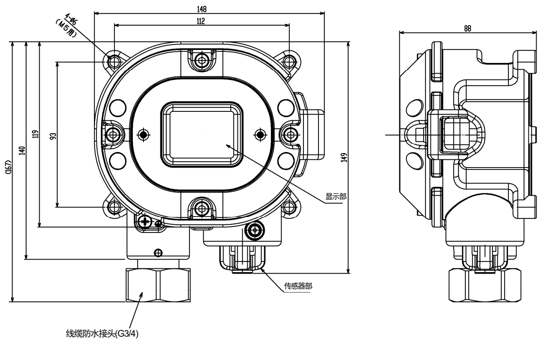
外观图
