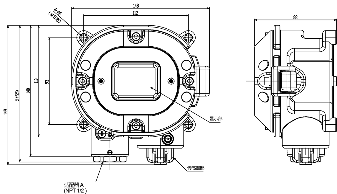
外观图
